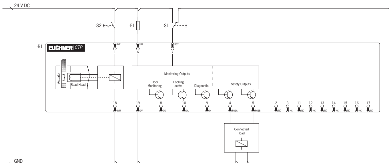
Obr. 3: Příklad připojení: Provedení s konektorem M23
