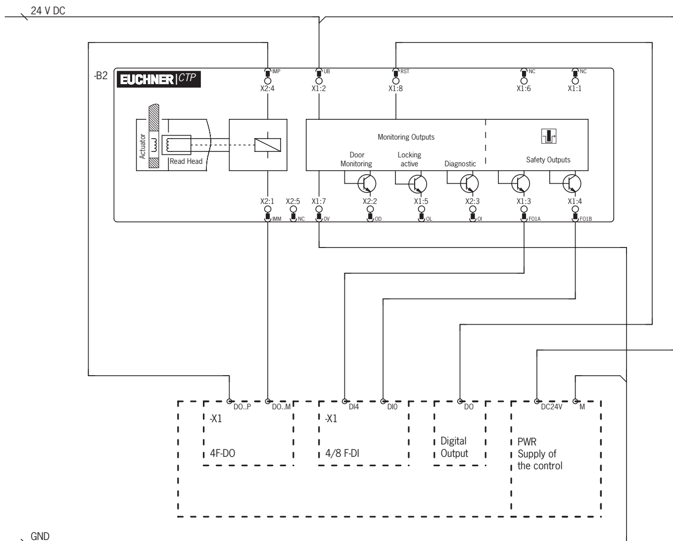
Obr. 4: Příklad připojení k systému ET200
