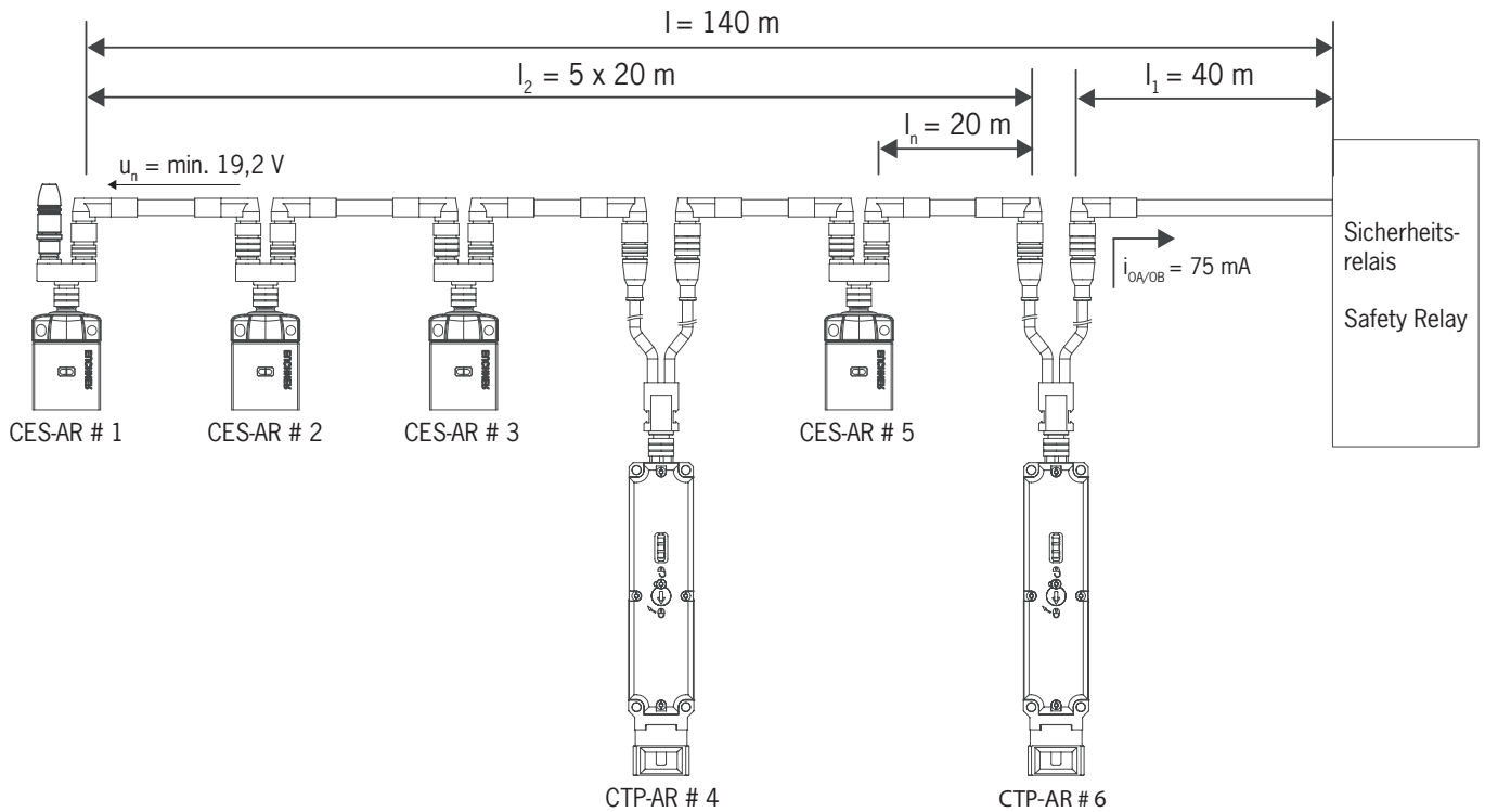
Figura 3: Ejemplo de conexión de seis interruptores CES-AR/CTP-L1-...
