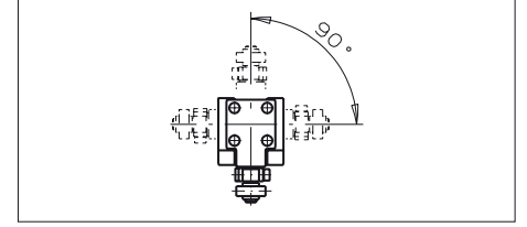
Resim 3: Yatay uygulanabilirlik
