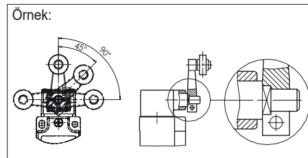
Resim 2: Aktüatörün dikey uygulanabilirliği
