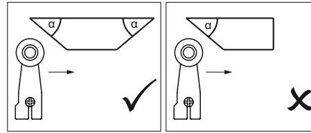
Resim 1: Kam şekli
