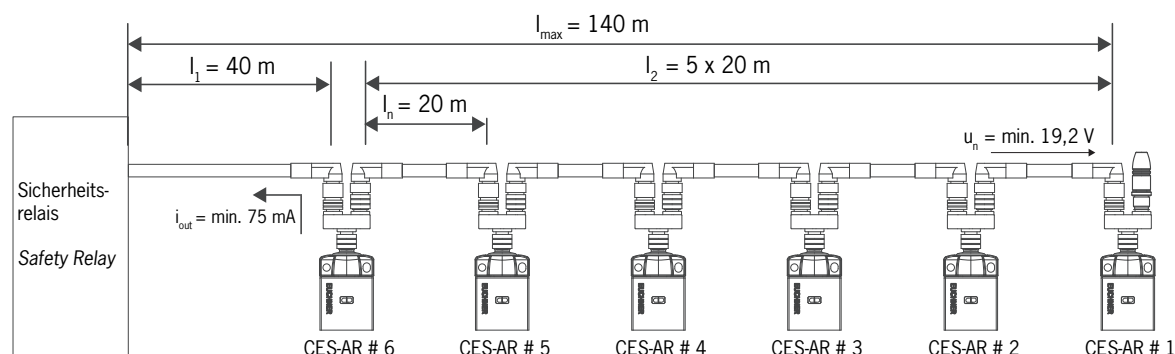
Figura 1: Ejemplo de conexión de seis interruptores CES-AR
