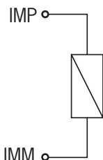
Obr. 7: Příklad připojení s přípojkou IMM
