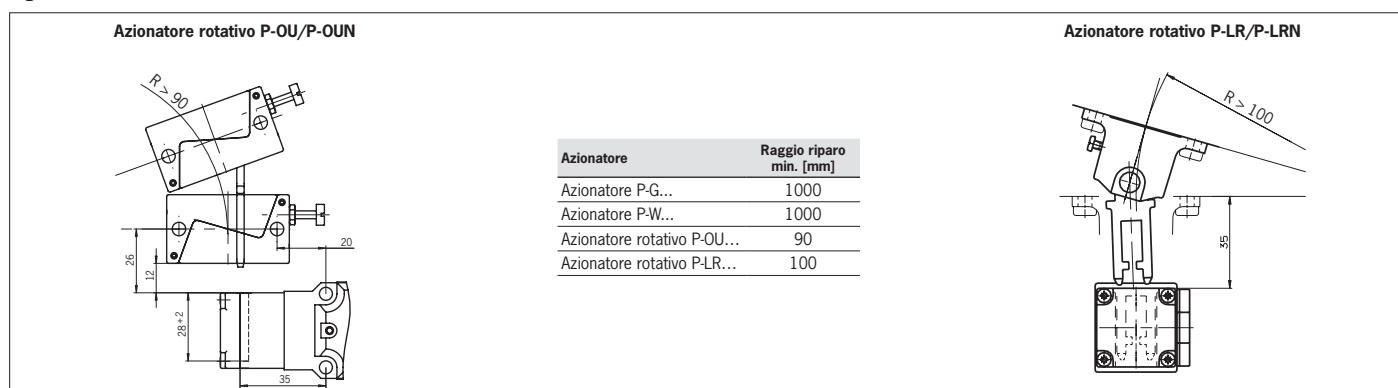
Figura 6: Raggi del riparo minimi
