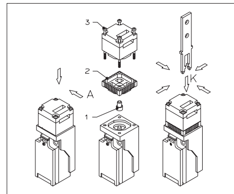
Figura 2: Installazione dell'adattatore NP-K
