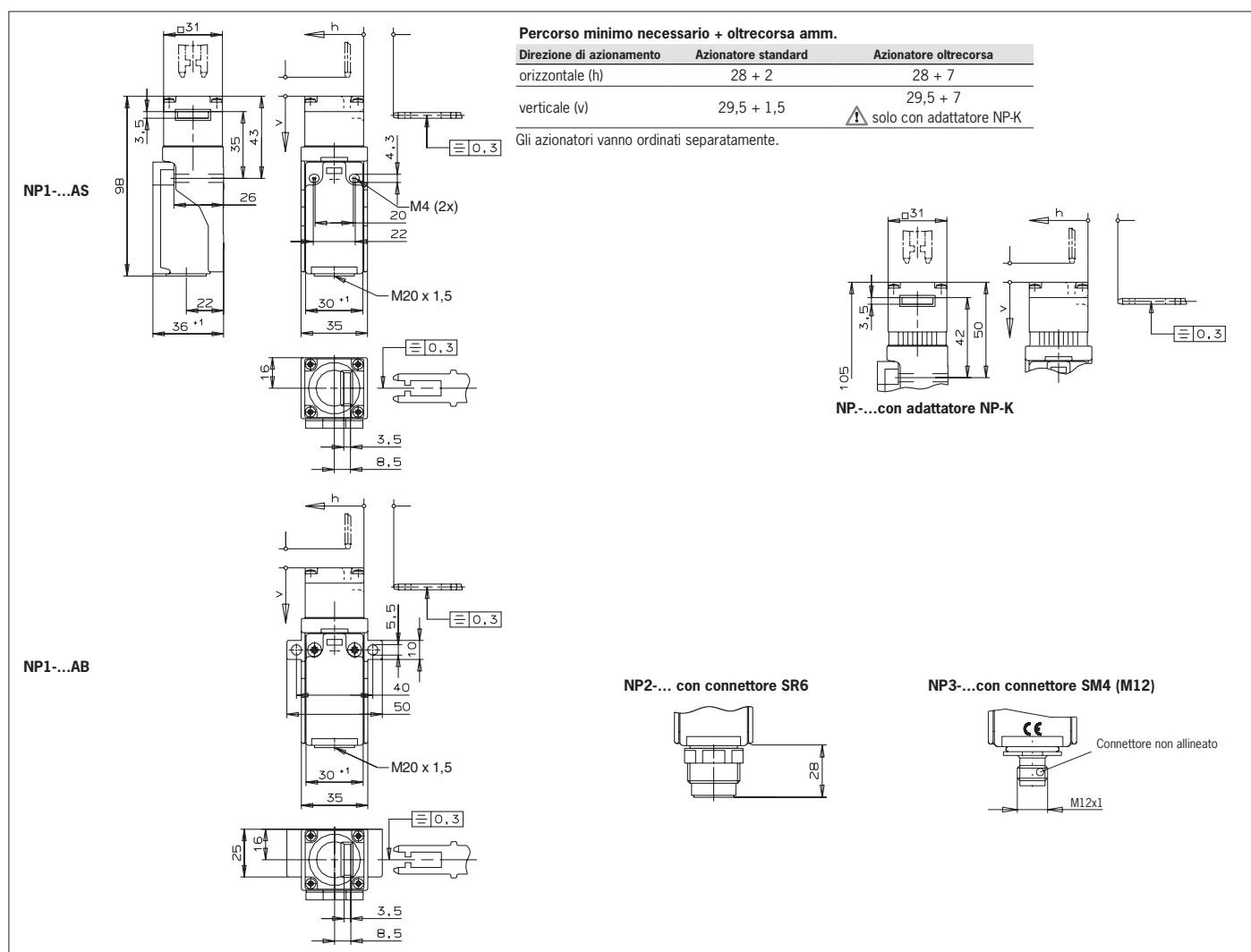
Figura 5: Dimensioni NP...
