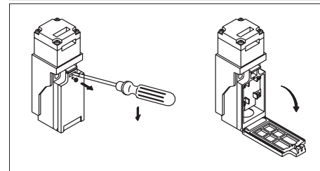
Figura 3: Apertura del finecorsa di sicurezza
