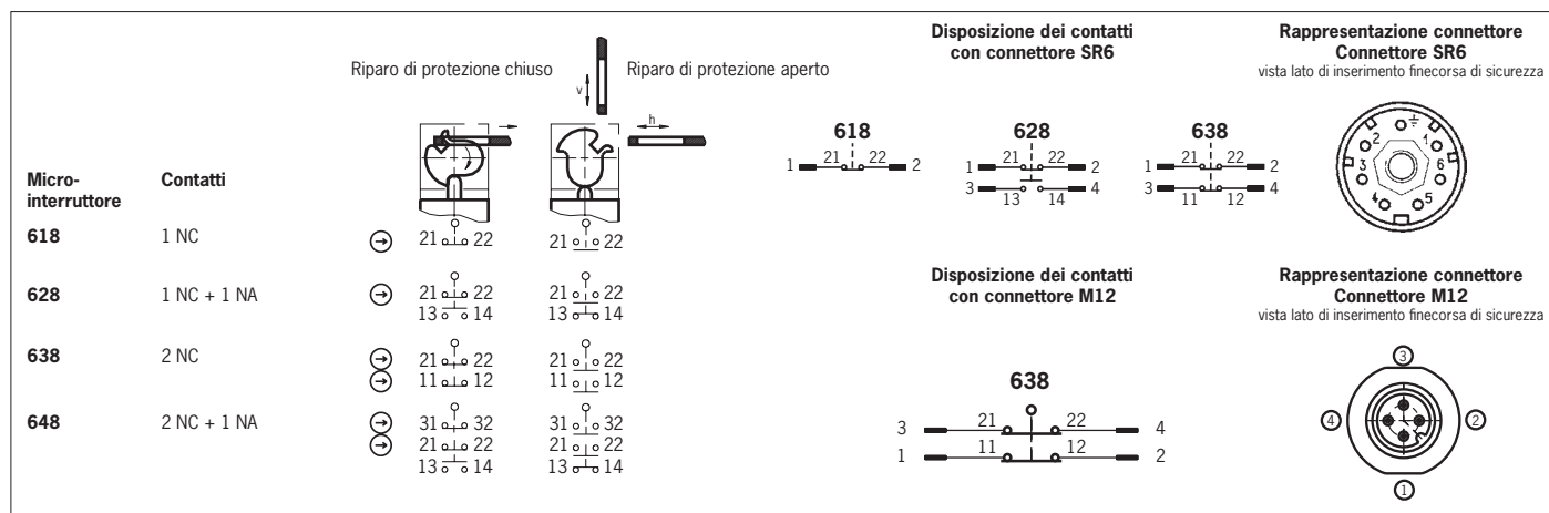
Figura 4: Microinterruttori e commutazioni
