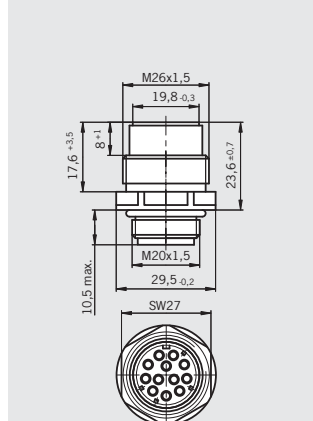
Vista del lado de conexión macho
