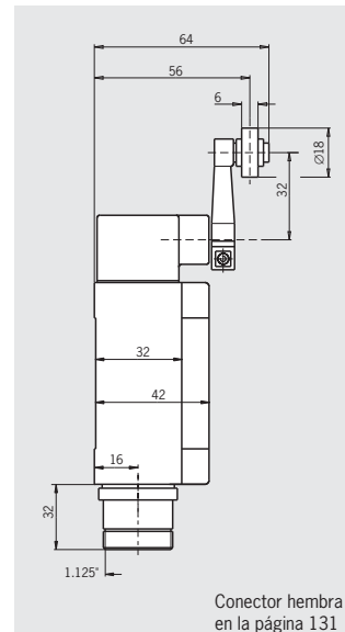
Conector MR9 8 polos + PE
