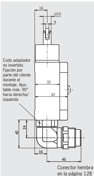
Conector SR6 acodado 6 polos + PE
