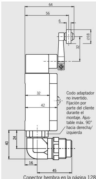
Conector SR6 acodado 6 polos + PE
