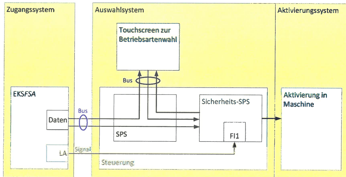
Abbildung 1: Prinzipschaltbild der Betriebsartenwahl
